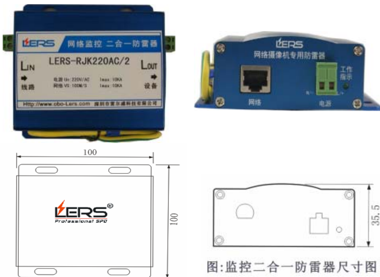
图: 监控二合一防雷器尺寸图
