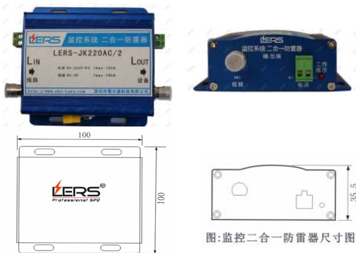
图:监控二合一防雷器尺寸图
